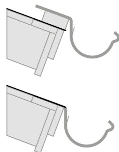
Hak długi
